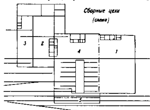
Фиг. 2. Сборные цехи Муромских мастерских: 1—механический; 2—котельный; 3—тендерный; 4—сборный; 5—малый.
