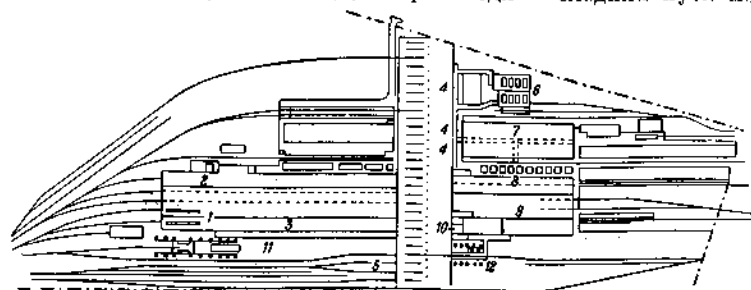
Фиг. 1. Мастерская в Декатуре (США): 1—место для заправки паровоза; 2—котельная; 3—тендерная; 4—машинная; 5—место для разборки паровоза; 6—силовая станция; 7—кузница; 8—колесоточная; 9—пригоночная; 10—распределительное бюро; 11—кран на 10 т; 12—кран на 5 т.
