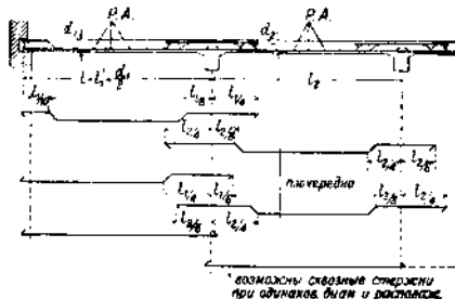
Фиг. 4. Перекрытия.
