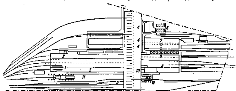
Фиг. 1. Мастерская в Денатуре (США): 1—место для заправки паровоза; 2—котельная; 3—тендерная; 4—машинная; 5—место для разборки паровоза; 6—силовая станция; 7—кузница; 8—колесоточарная; 9—пригоночная; 10—распределительное бюро; 11—кран на 10 т; 12—кран на 5 т.
