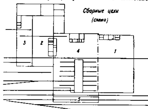
Фиг. 2. Сборные цехи Муровских мастерских: 1—механический; 2—котельный; 3—тендерный; 4—сборный; 5—маллярный.
