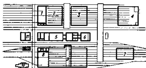
Фиг. 4. Вагоносборная мастерская: 1—токаря; 2—сборная пассаж. ваг.; 3—маллярная; 4—сборная пассаж. ваг.; 5—кузница; 6—столярная; 7—маллярная тон. ваг.; 8—деревосборная; 9—сборная тон. ваг.; 10—контора; 11—силовая станция.
