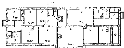
Фиг. 1. 1—табеляная, 2—жилые комнаты, 3—столовая, 4—спальня, 5—кухня, 6—умывальная, 7—уборная, 8—кладовая, 9—сени, 10—раздевальня, 11—сушильный шкаф.
